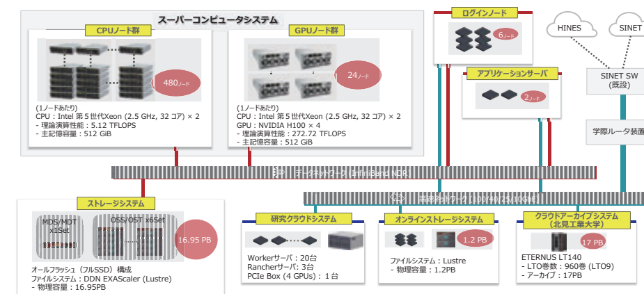
新学際大規模計算機システムの構成図
