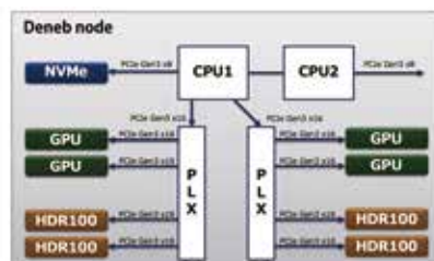
図2 Albireo nodeとDeneb nodeのブロックダイアグラム
