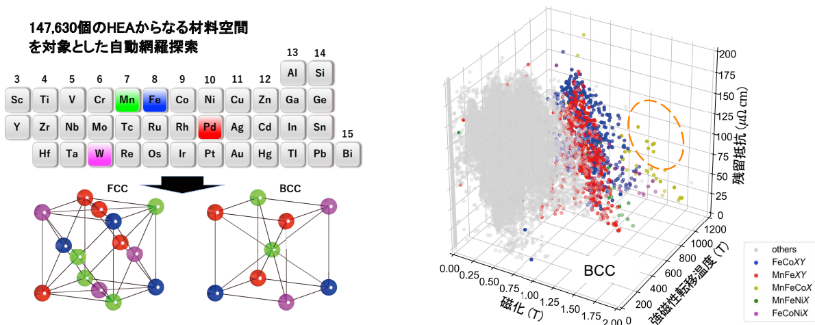
図1. (左) 面心立方格子 (FCC) と体心立方格子 (BCC) を有する 4 元高エントロピー合金 (HEA) から成る材料空間 (合計 147,630 個)。例として Mn、Fe、Pd、W が記されている。 (右) 「富岳」と「AkaiKKR」による自動網羅計算の結果 (BCC の場合のみ)。各軸は磁化、強磁性転移温度、残留抵抗に対応する。オレンジ色の領域は高性能軟磁性材料として有望な系である。
